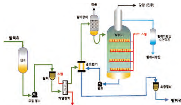
[그림 5] 식용유 탈취 공정 장치 간략 공정도
